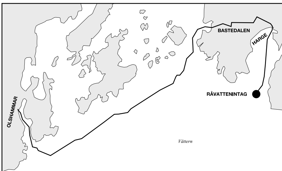
Sjöförlagd vattenledning mellan Harge och Olshammar via Bastedalen.
